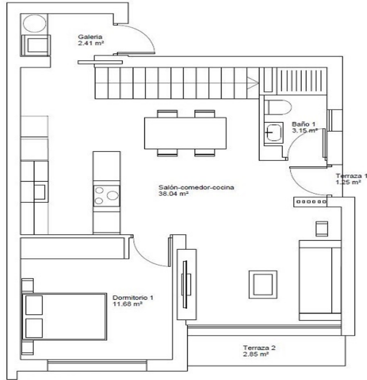
PLANO PLANTA BAJA
